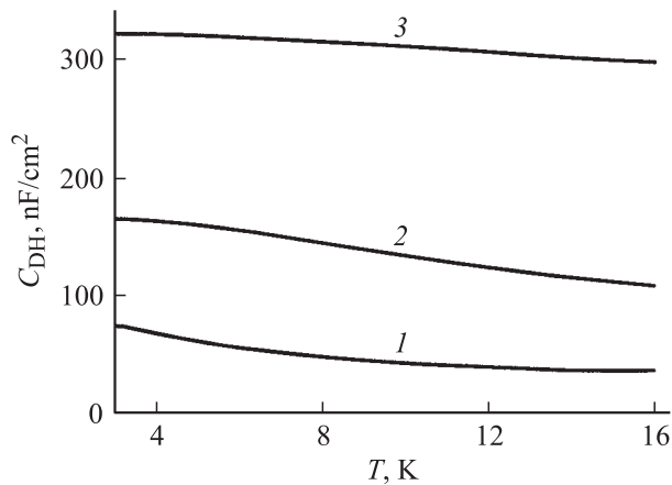
Рис. 2. Температурная зависимость емкости \varepsilon/\Lambda_{\text{ДН}} , приходящейся на единицу плоской поверхности p\text{-Si:B} , при |e\varphi_s| \ll k_B T для концентрации N = 10^{17} \text{ см}^{-3} при различных степенях компенсации K атомов бора: 1 – 10^{-4} , 2 – 10^{-3} , 3 – 10^{-2} .
