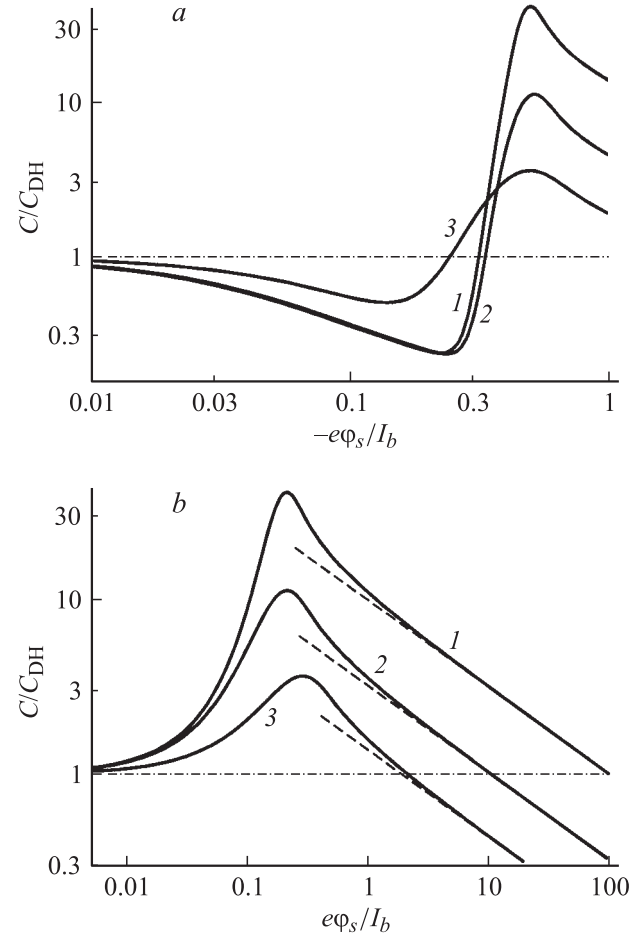
Рис. 1. Зависимость квазистатической емкости C кристалла p\text{-Si:B} от отрицательного (а) и положительного (б) электростатического потенциала \varphi_s на поверхности для N = 10^{17} \text{ см}^{-3} при T = 10 \text{ К} и степенях компенсации K : 1 — 10^{-4} , 2 — 10^{-3} , 3 — 10^{-2} . Штриховые линии — емкость в режиме Шоттки–Мотта C_{SM}/C_{DH} = \Lambda_{DH}/\Lambda_{SM} .
