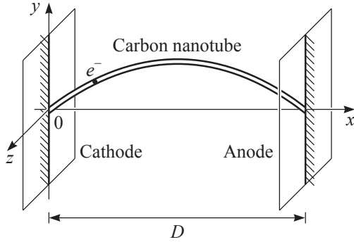
Рисунок 1 – Электрон ( e^- ) внутри полый углеродной нанотрубки длиной L , сжатой между катодом ( x = 0 ) и анодом ( x = D ) и выгнутой в плоскости xy
