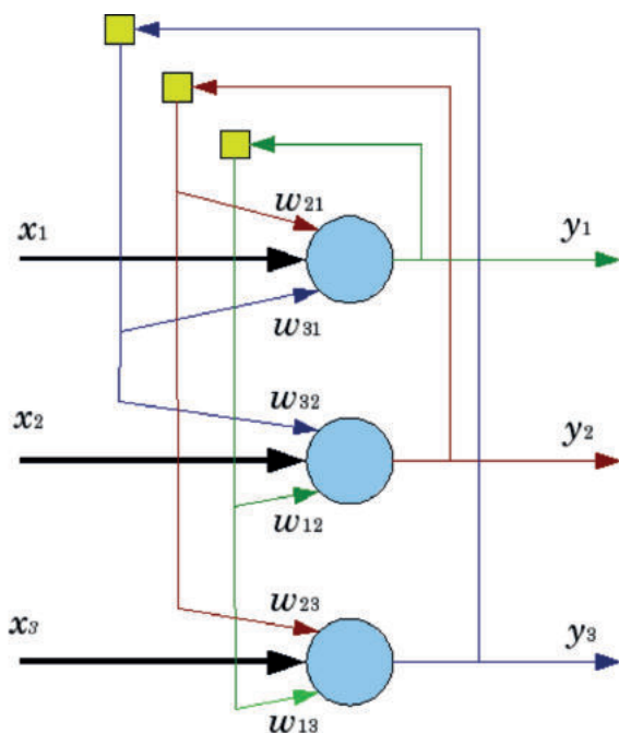
Рис. 9. Архитектура нейронной сети Хопфилда
