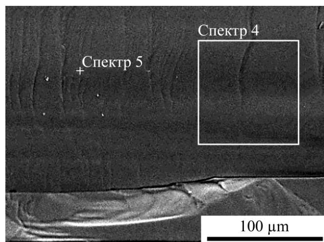
Рис. 1. Скопления примесных атомов никеля в образцах Si<Ni>.
