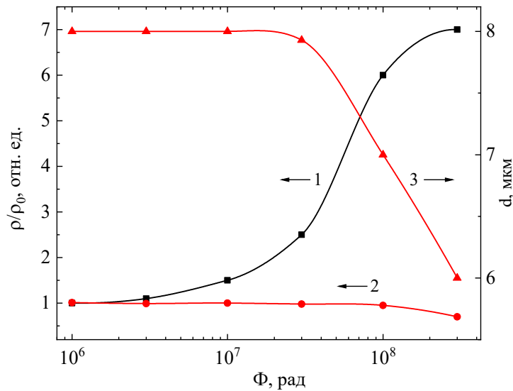
Рис. 3. Относительное изменение удельного сопротивления контрольных образцов кремния (1) и Si<Ni> (2) от дозы \gamma -облучения, (3) изменение размеров скоплений от дозы \gamma -облучения.
