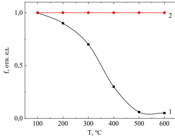
Рис. 4. Отжиг радиационных дефектов в контрольных образцах кремния (1) и в Si<Ni> (2).
