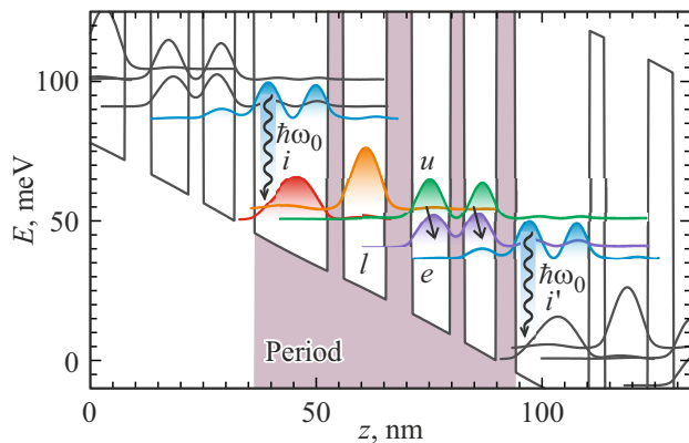
Рис. 1. Диаграмма зоны проводимости и квадраты модулей волновых функций электронов исследуемого ККЛ, рассчитанные \mathbf{k} \cdot \mathbf{p} -методом при температуре T = 55 К и напряжении на периоде структуры V = 50 мВ. Прямые стрелками показаны излучательные переходы, \hbar\omega_0 — энергия продольного оптического фонона.
