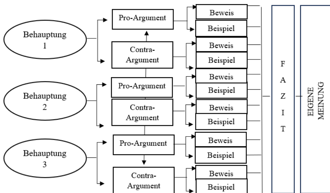
Технология аргумент-картирования
