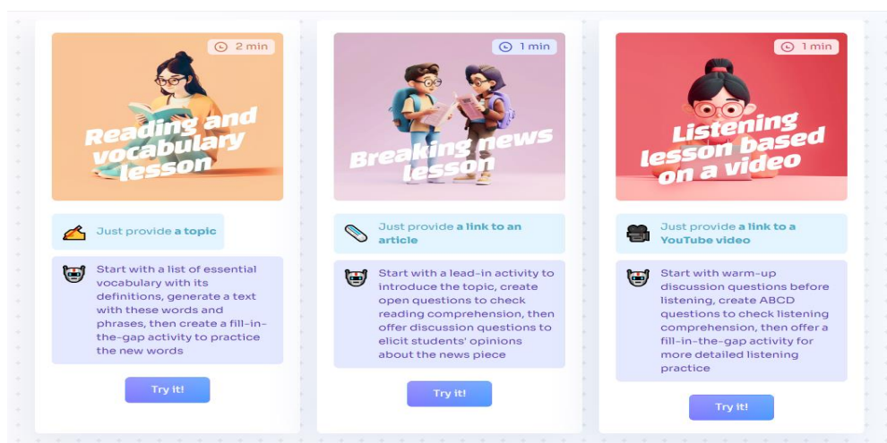
Рис. 1. Опции платформы
