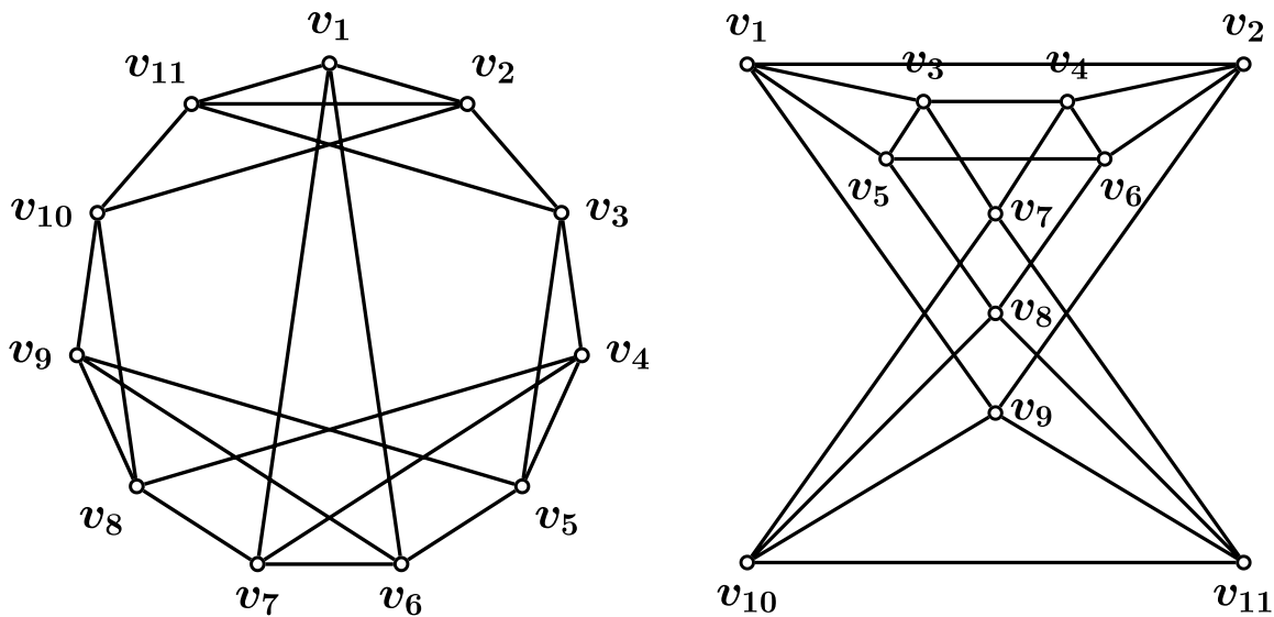
Регулярный граф четвертой степени с одиннадцатью вершинами, в котором между любыми двумя вершинами существует путь длины два
