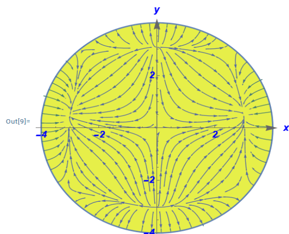
Рис. 4. Визуализация электрического поля.
