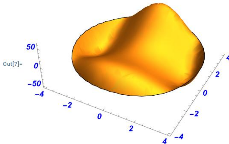
Рис. 3. Визуализация решения в трехмерном пространстве.
