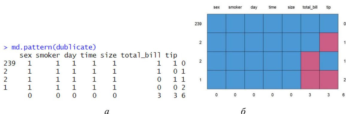
Рис. 3. Пример работы функции md.pattern() : a – табличное представление; б – матричная визуализация
