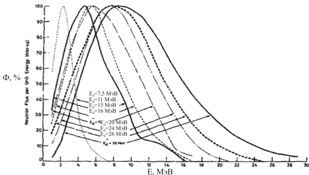
Рисунок 2 – Относительные спектры нейтронов, вылетевших под углом 0^\circ из толстых мишеней Ве, бомбардированных дейтронами [3]
