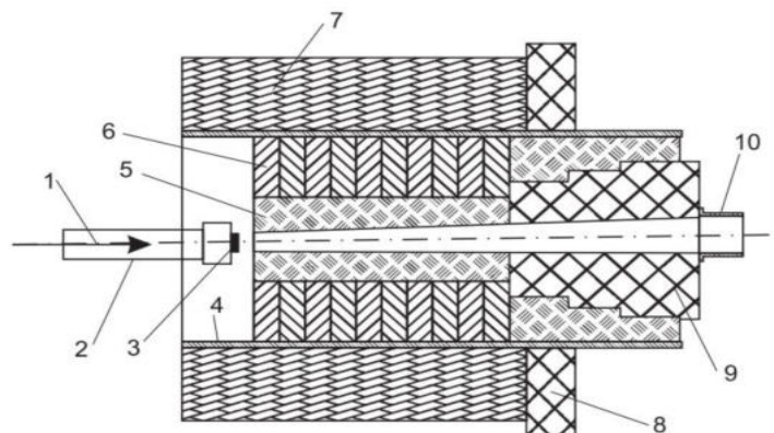
Рисунок 1 – Коллиматор нейтронного пучка: 1 – пучок дейтронов; 2 – канал ионного пучка; 3 – Ве-мишень; 4 – железная труба; 5 – полиэтиленовый коллиматор; 6 – железные диски; 7 – бетонная стена; 8 – радиационная защита из полиэтилена; 9 – съемный полиэтиленовый коллиматор; 10 – конус
