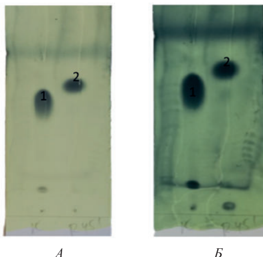
Рисунок 2 – ТСХ контроль-реакционная смесь через 45 мин после начала метанолиза пальмового (А) и кокосового (Б) масел: 1 – образец растительного масла, 2 – метиловые эфиры ЖК.
