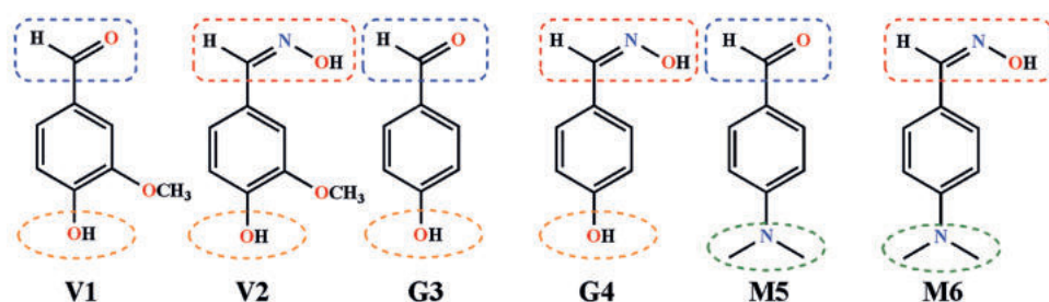
Рисунок 4 – Структурные формулы исследуемых соединений
