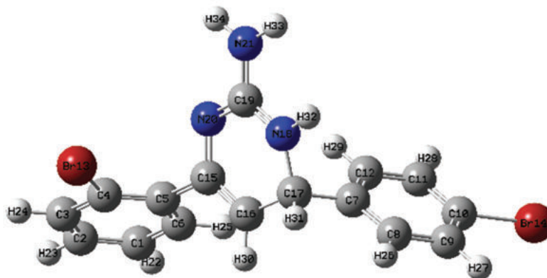
Рисунок 1 – Оптимизированная молекула методом РМ6
