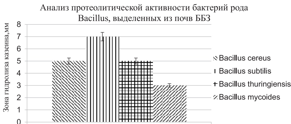
Рисунок 3 – Анализ протеолитической активности бактерий рода Bacillus , выделенных из почв ББЗ
