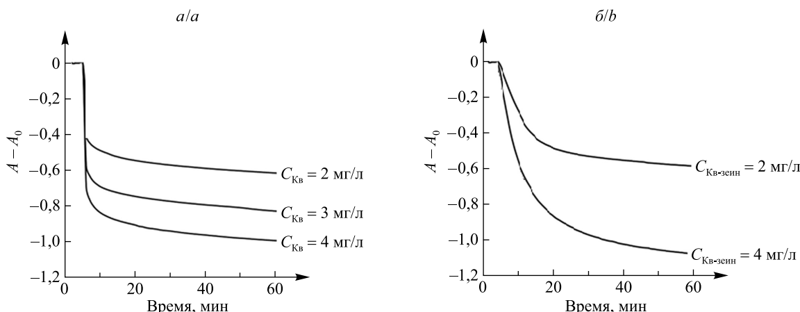
Рис. 1. Кинетические кривые обесцвечивания растворов катион-радикалов АБТС нативным кверцетином (а) и кверцетином, включенным в наночастицы зеина (б). Концентрации нативного ( C_{KB} ) и наноструктурированного ( C_{KB-зеин} ) кверцетина указаны на рисунке, концентрация катион-радикалов АБТС составляет 8,7 \cdot 10^{-5} моль/л, температура – 20 °С, длина волны – 734 нм
