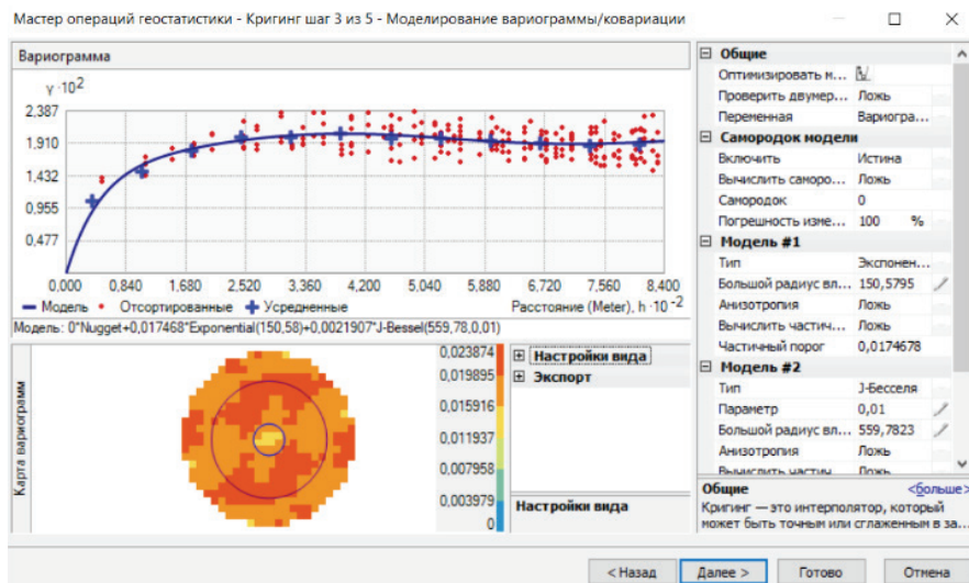
Рис.4. Теоретическая вариограмма
