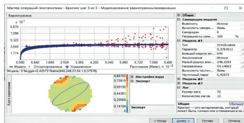
Рис. 3. Теоретическая вариограмма
