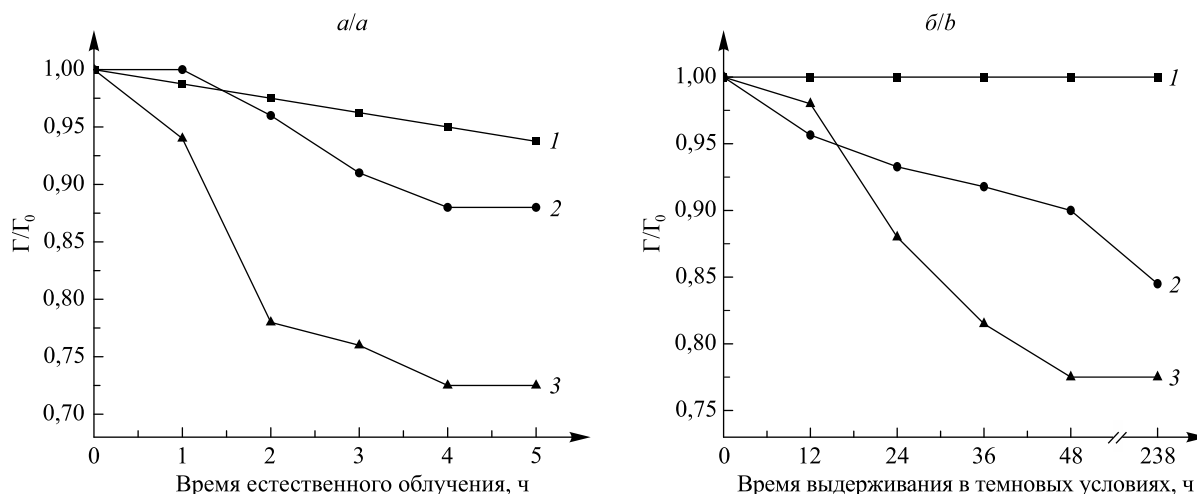
Рис. 2. Относительное изменение поверхностной концентрации родамина 6G на световых (а) и темновых (б) временных промежутках на рис. 1 для пленочных фотокатализаторов TiO 2 (1), TiO 2 :NiHPM (2), TiO 2 /MoO 3 (3)
