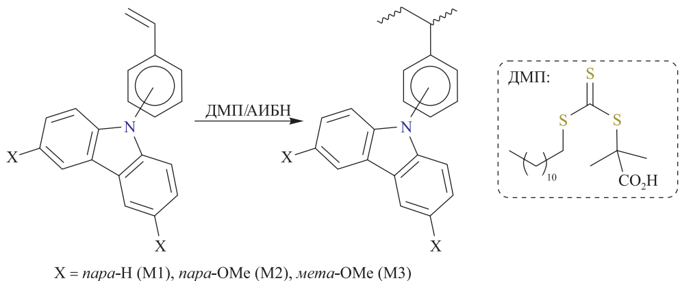
Рис. 1. Схема RAFT-полимеризации карбазолсодержащих мономеров стирольного типа M1 – M3 на иницирующей системе ДМП/АИБН
