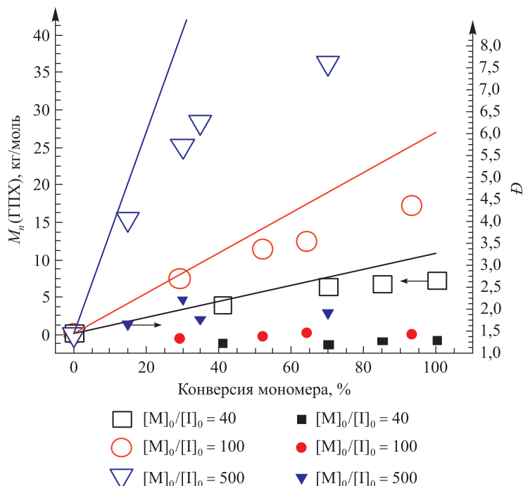
Рис. 5. Графики зависимости M_n (ГПХ) и D от конверсии мономера для RAFT-полимеризации мономера M1 на иницирующей системе ДМП/АИБН при температуре 70 °С в циклогексаноне при различных соотношениях [M]_0/[I]_0 .
