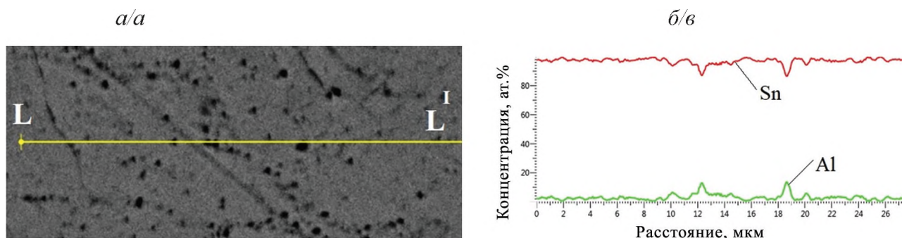
Рис. 2. Микроструктура а и распределение Al и Sn вдоль линии сканирования L–L 1 фольги сплава Al – 96,7 ат. % Sn
