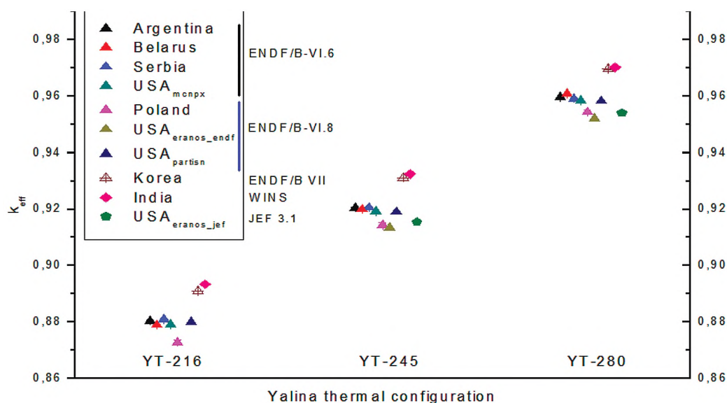
Рис. 8. Зависимость эффективного коэффициента размножения k_{eff} для ПКС «ЯЛНА-Тепловая» от количества загруженных ТВЭЛов
