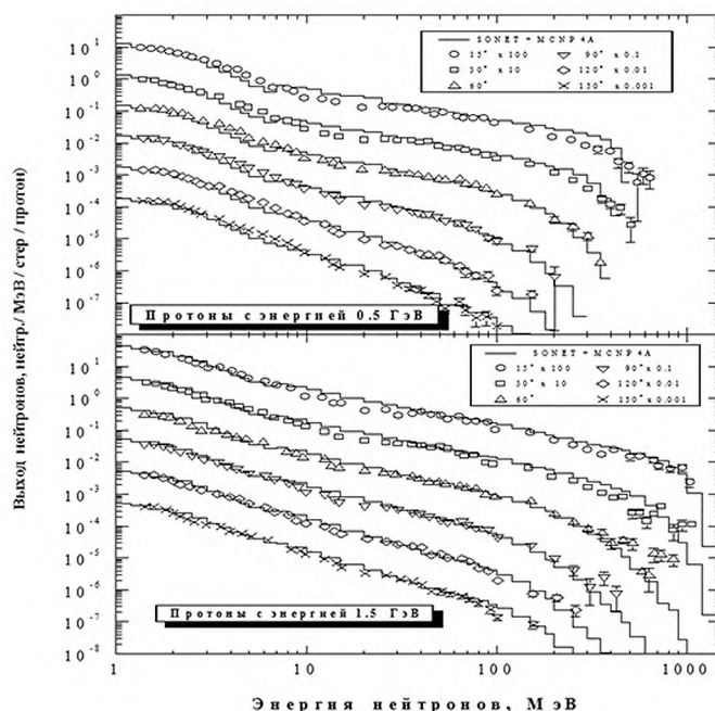
Рис. 1. Экспериментальные и расчетные спектры нейтронов, вылетающих из свинцовой мишени 15 \times 15 \times 20 см 3 , при облучении протонами с энергией 0,5 и 1,5 ГэВ. Гистограммы – расчеты по SONET+MCNP4A [11], символы – экспериментальные данные [12]
