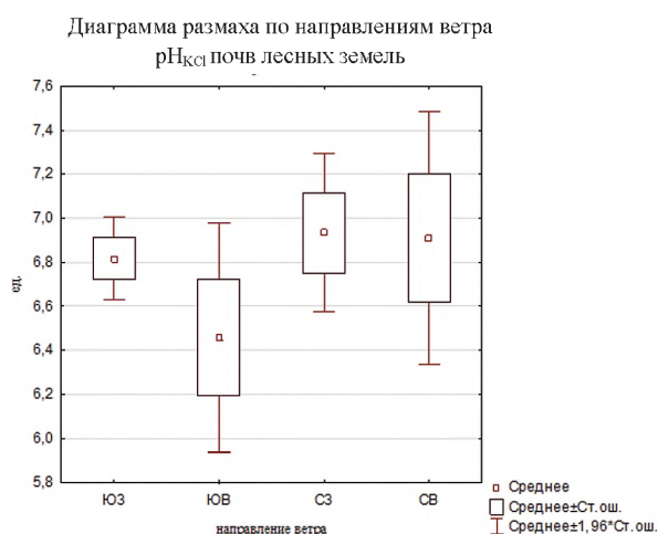
Рис. 2. Диаграмма размаха средних значений pH_{KCl} почв лесных земель по направлениям ветра
