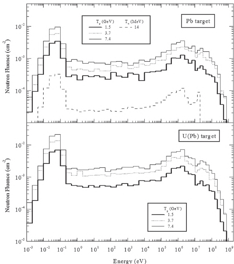
Рис. 4. Рассчитанные энергетические спектры нейтронов, усредненные по объему Ла-образца (№ 3) в системе «Pb и U(Pb)-замедлитель», для протонных и нейтронных пучков. Данные нормированы на одну частицу первичного пучка
