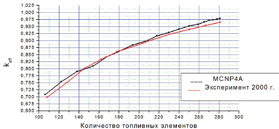
Рис. 6. Зависимость эффективного коэффициента размножения ПКС «ЯЛИНА-Тепловая» от количества загружаемых топливных элементов: расчеты по MCNP 4A; экспериментальные данные
