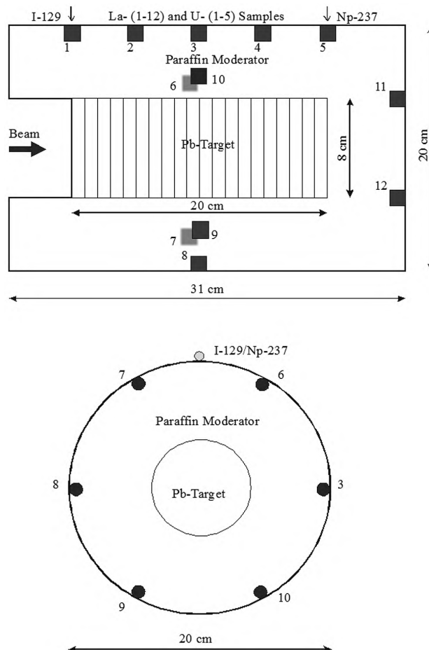
Рис. 3. Схема расположения образцов из Np, I, La в свинцово-парафиновой мишени, облучаемой протонами с энергиями 1,5 ГэВ; 3,7 ГэВ и 7,4 ГэВ
