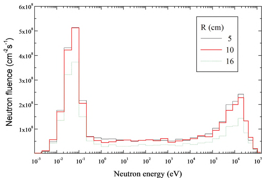
Рис. 5. Плотность потока нейтронов в экспериментальных каналах уран-полиэтиленовой подкритической сборки, управляемой генератором нейтронов. Интенсивность генератора нейтронов в расчетах принята 10^{12} нейтр./с
