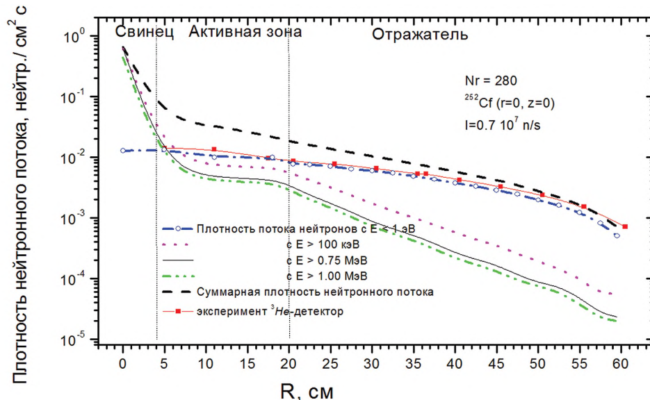
Рис. 7. Радиальное распределение плотностей потока нейтронов в канале EC1 (R=5 см) ПКС «ЯЛИНА-Тепловая» для ^{252}\text{Cf} -источника: --- нейтроны с E_n > 0,75 МэВ; -.-.- нейтроны с энергией < 1 эВ; ..... нейтроны с энергией > 100 эВ; ..... – нейтроны всех энергий; ■ – экспериментальные данные, измеренные ^3\text{He} -детектором
