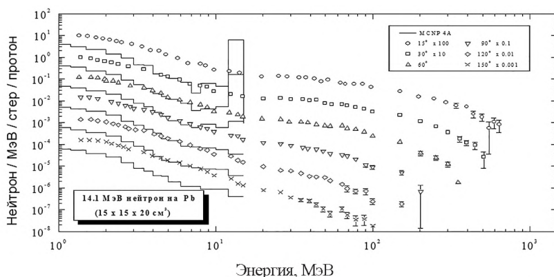
Рис. 2. Экспериментальные и расчетные спектры нейтронов, вылетающих из свинцовой мишени 15 \times 15 \times 20 \text{ см}^3 , при облучении нейтронами с энергией ~14 МэВ. Гистограммы – расчеты по SONENT+MCNP4A [11], символы – экспериментальные данные [12]
