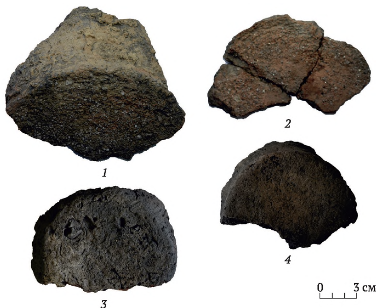
Рис. 5. Фрагменты сосудов со следами подсыпки на дне (1-2 – дресва; 3 – полова; 4 – древесная зола) (фотографии В. Н. Бахматовой) Fig. 5. Fragments bottoms of vessels with traces from the filling (1-2 – the broken stone; 3 – the husks from grains; 4 – the wood ash) (photos by V. N. Bakhmatova)
