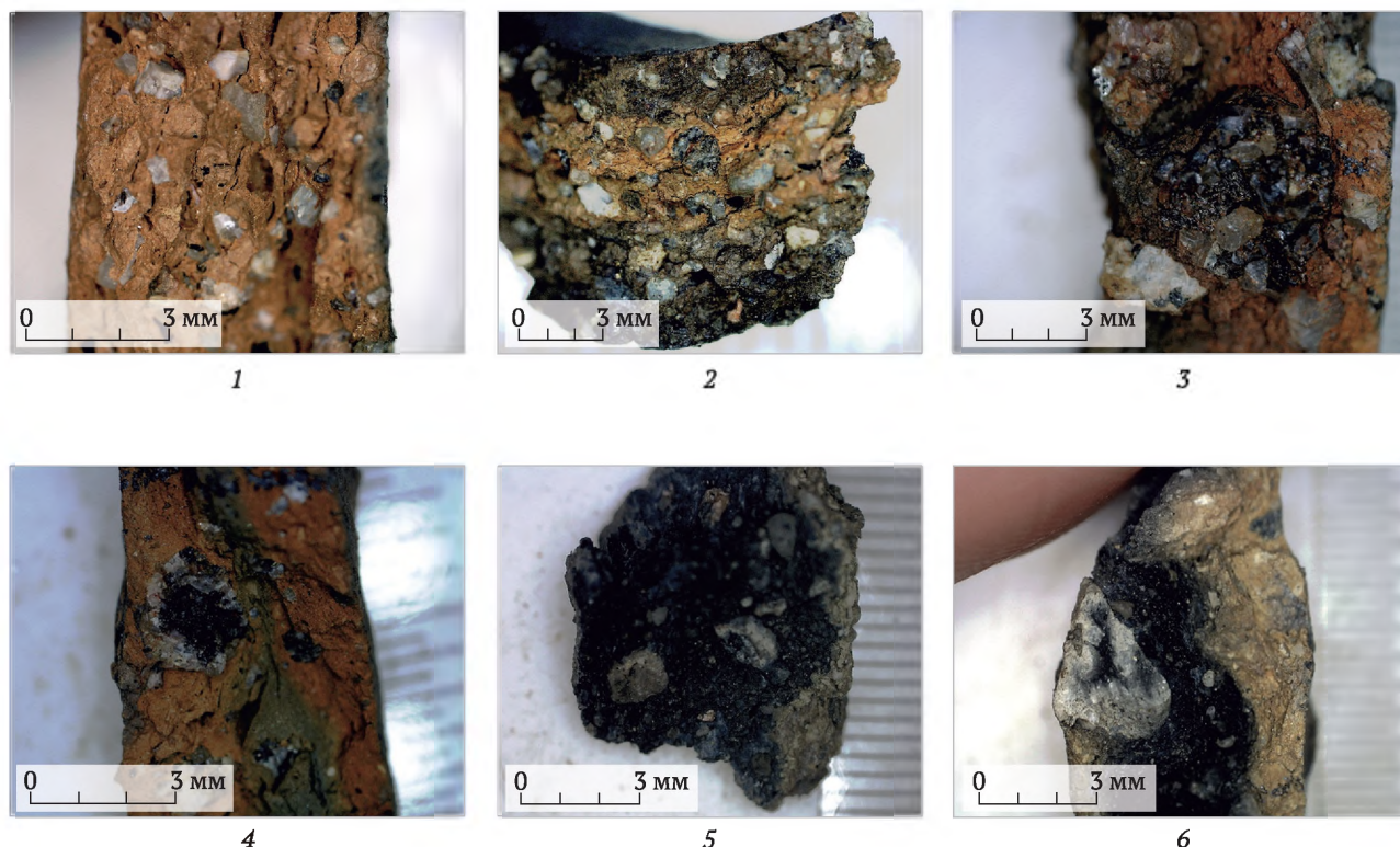
Рис. 3. Изломы сосудов с минеральными примесями в составе формовочной массы (1–4 – дресва; 5 – дресва и песок; 6 – шамот и песок) (фотографии В. Н. Бахматовой)
