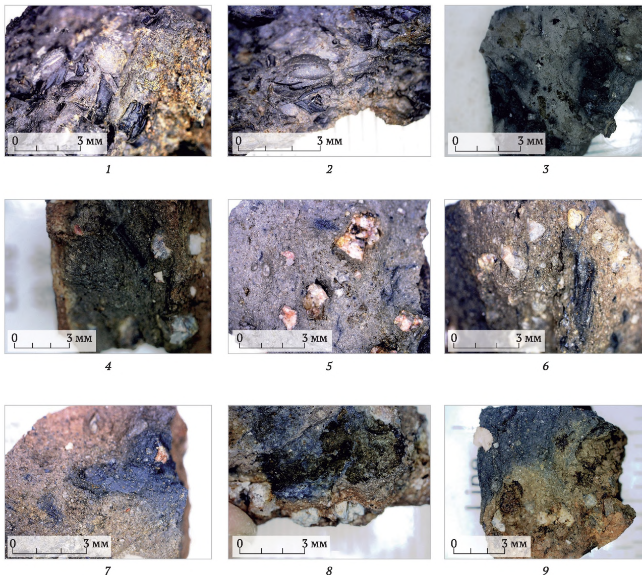
Рис. 4. Изломы сосудов с органическими примесями в составе формовочной массы (1–3 – отходы от обмолота зерновых культур; 4–6 – выжимка из навоза; 7–9 – органический раствор) (фотографии В. Н. Бахматовой)
