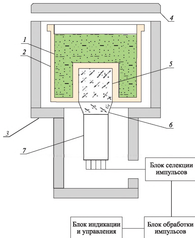
Рис. 3. Упрощенная функциональная схема гамма-радиометра РУГ-91М «Адани»:
