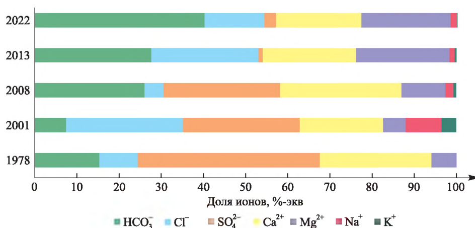
Рис. 4. Динамика показателей относительного содержания главных ионов в воде оз. Бредно с 1978 по 2022 г.
