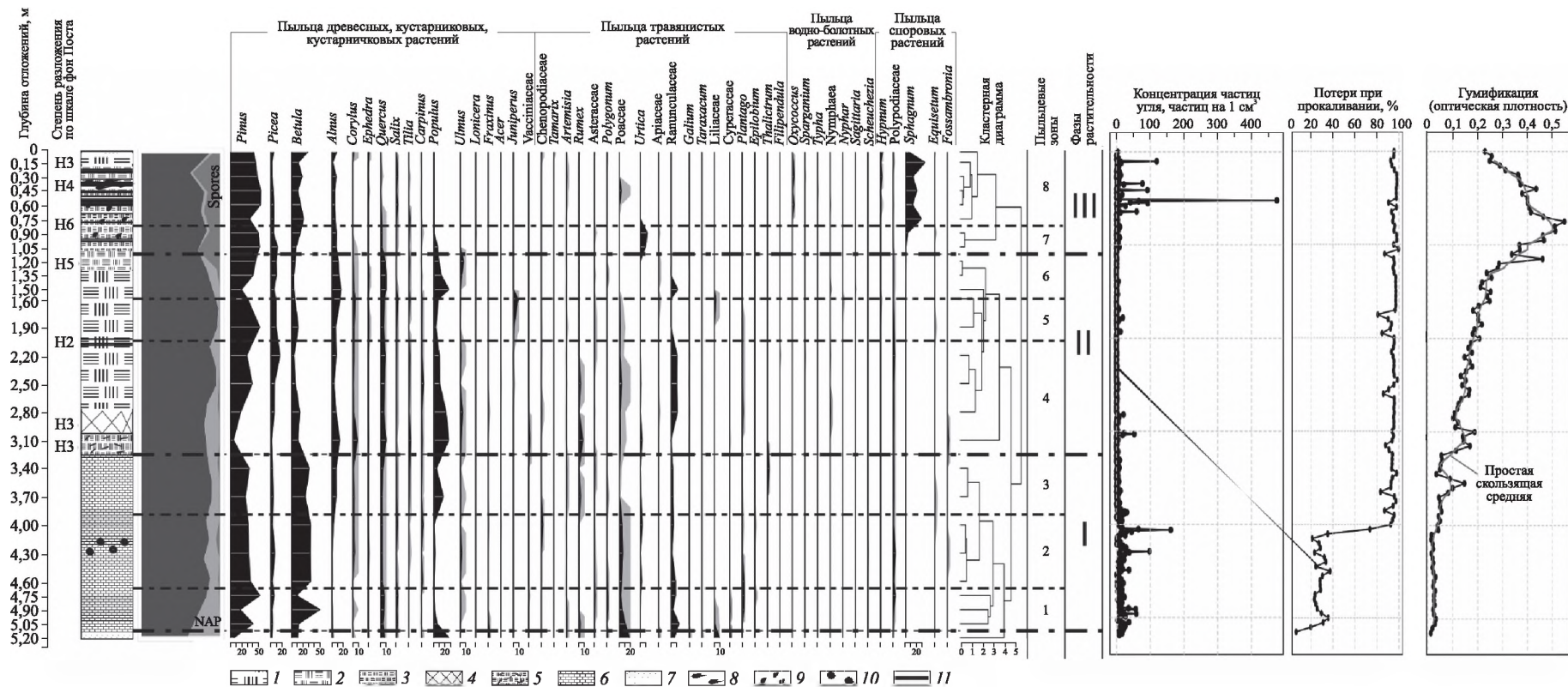
Рис. 2. Отложения болота Шкреды:
