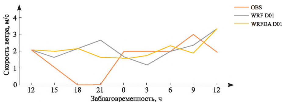
Рис. 3. Прогноз скорости приземного ветра на высоте 10 м, м/с: OBS – наблюдения на станции Мозыря; WRF D01 – без ассимиляции; WRFDA D01 – с ассимиляцией. 26.01.2019 г.
