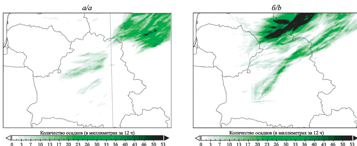
Рис. 4. Карта распределения осадков (в миллиметрах за 12 ч): a – с ассимиляцией данных (AS); b – без ассимиляции (NA). 02.08.2017 г.
