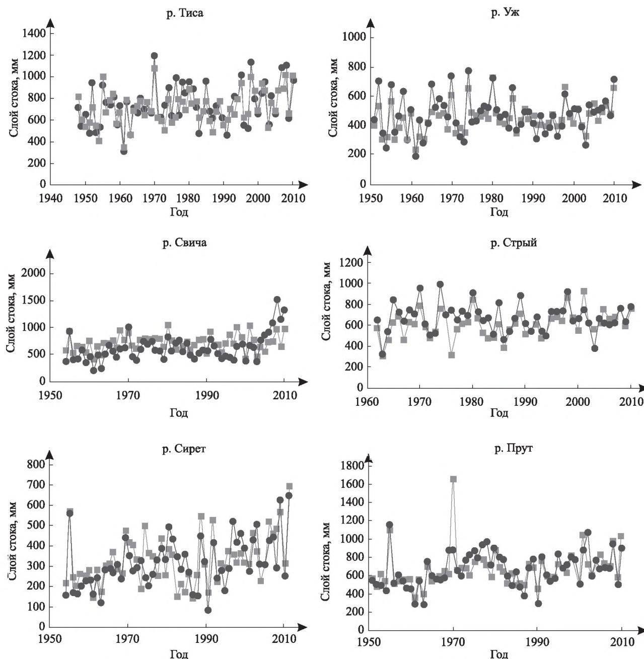
Рис. 2. Результаты сравнения фактических значений среднего годового слоя стока воды ( Qa_{\text{факт}} — ●—) исследуемых рек со смоделированным ( Qa_{\text{прогн}} — ■—)
