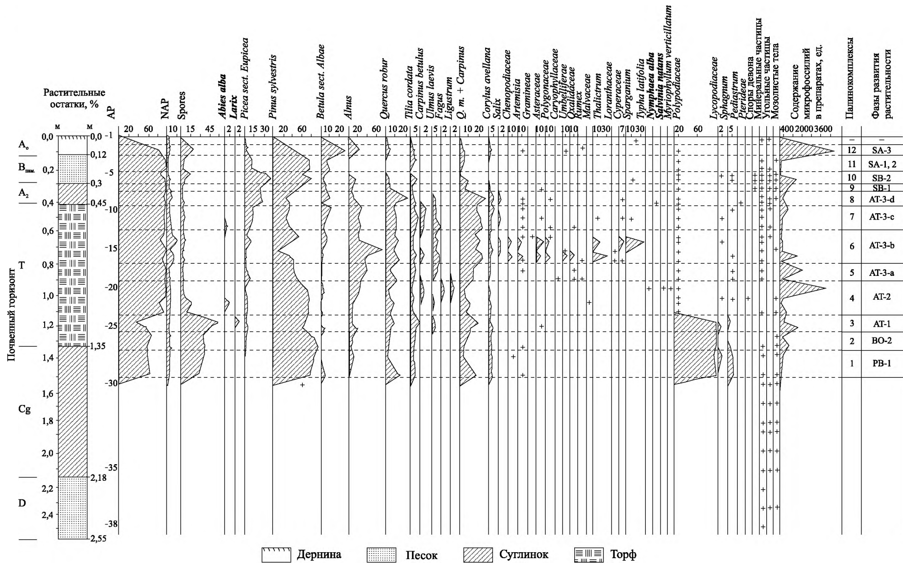
Рис. 1. Палинологическая диаграмма отложений в разрезе у д. Стайки (расчистка 2): PB – пребореальный; BO – бореальный; AT – атлантический; SB – суббореальный; SA – субатлантический периоды (анализ Я. К. Еловичевой по материалам Т. Н. Белоусовой)
