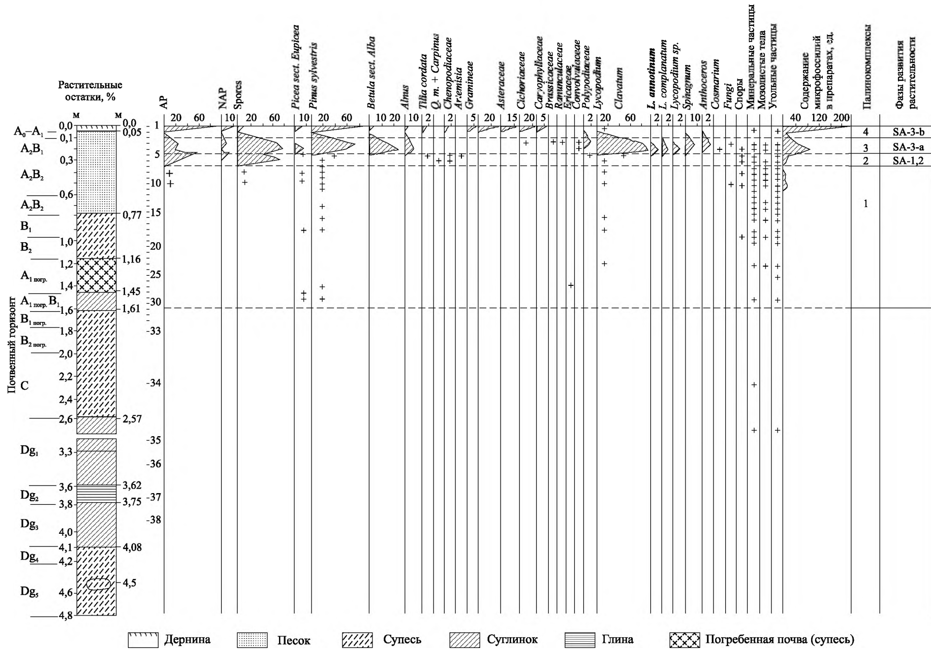
Рис. 2. Палинологическая диаграмма отложений в разрезе у д. Стайки (расчистка 1) (анализ Я. К. Еловичевой по материалам Т. Н. Белоусовой) Fig. 2. Palynological diagram of the deposits in the section near the vil. Stajki (clearing 1) (analysis by Y. K. Yelovicheva on the materials by T. N. Belousova)
