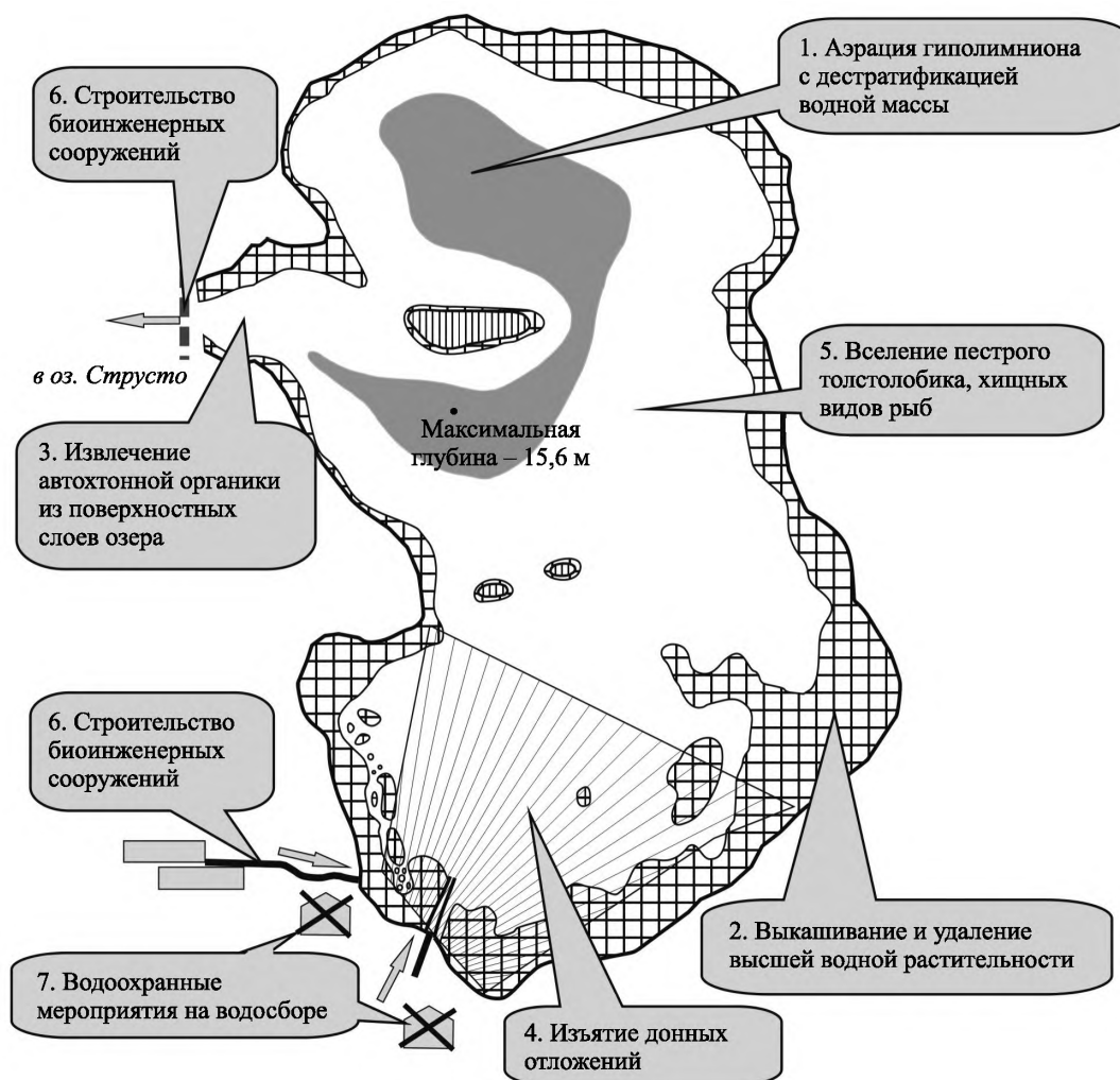
Рис. 7. Принципиальная схема технологии восстановления оз. Болойсо
