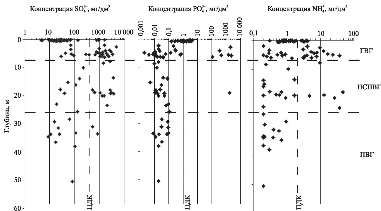
Рис. 2. Распределение загрязняющих веществ в зонах аэрации и водоносных горизонтов: ГВГ – грунтовый; НСПВГ – нижне-среднеплейстоценовый; ПВГ – палеогеновый
