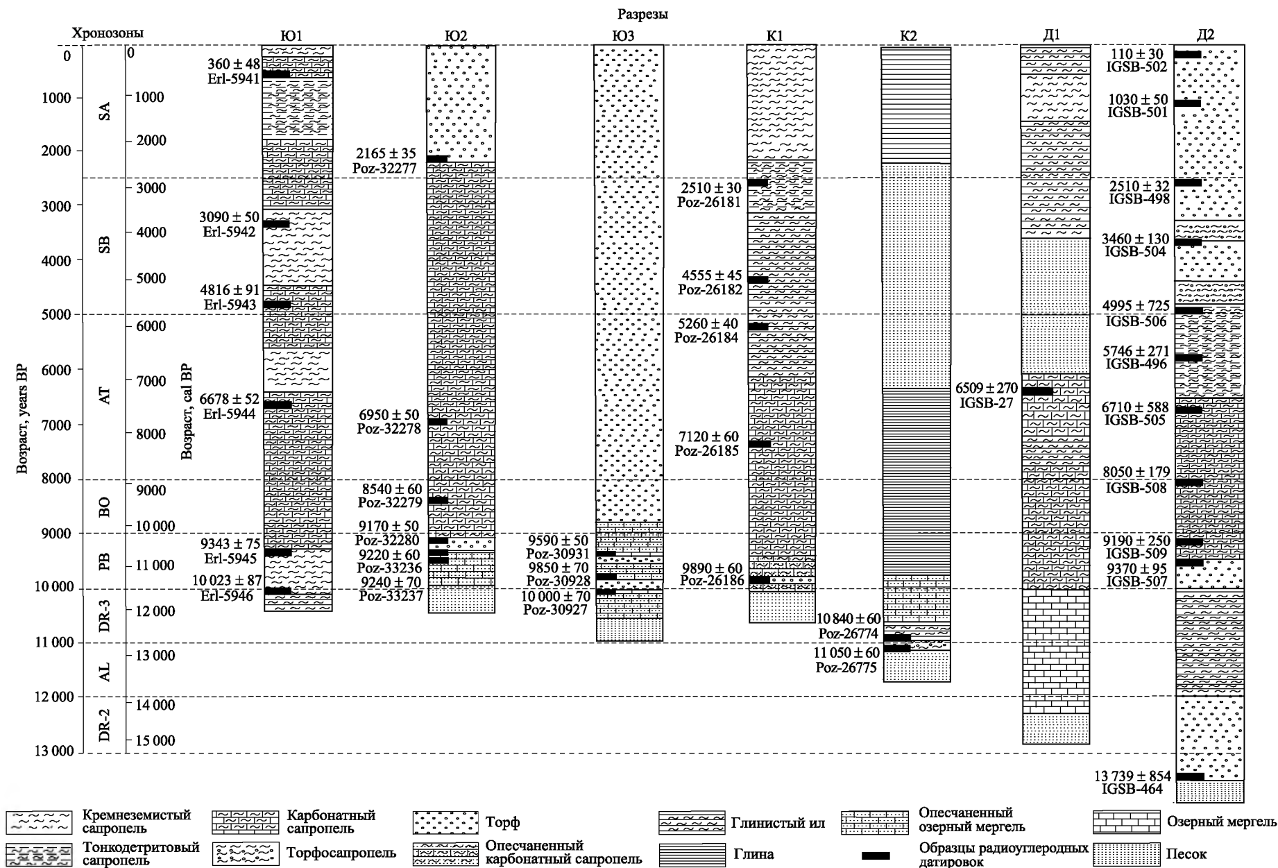
Рис. 2. Сравнительная литостратиграфия озерных осадков в регионе Балтийских Поозерий Fig. 2. Comparative lithostratigraphy of the investigated sediments in the Baltic Lake Districts
