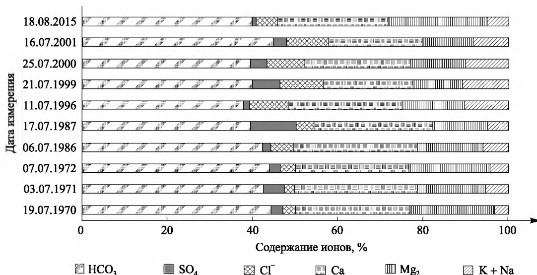
Рис. 3. Многолетняя динамика ионов в оз. Болойсо, %-экв
