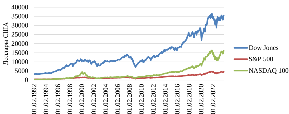
Рис. 1. Тенденции цен закрытия международных индексов, в долл. США
