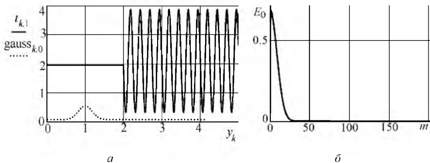
Рис. 1. Зонд вне объекта, объект (а) и результирующий спектр (б)
