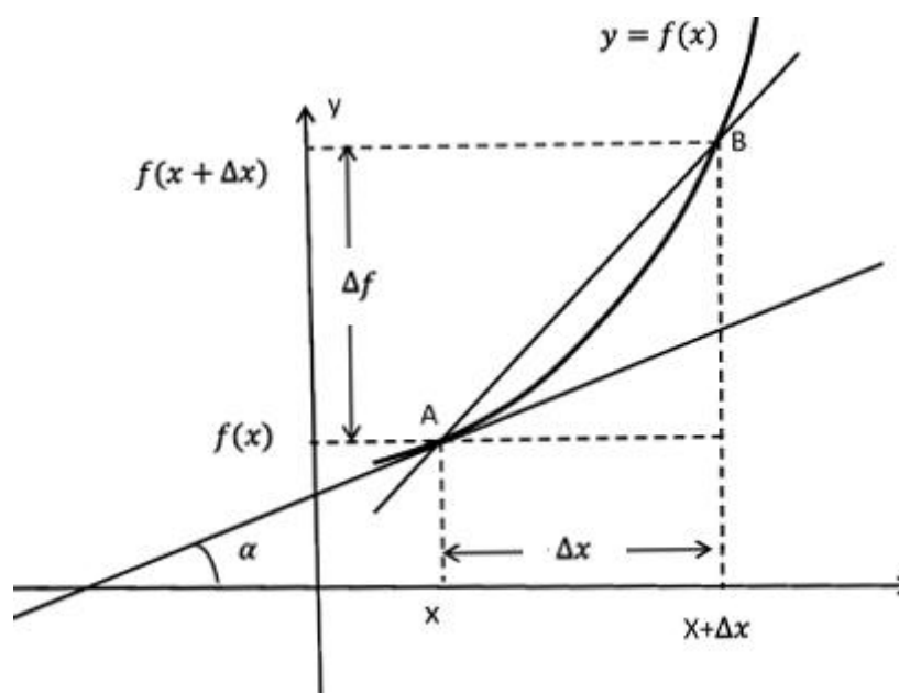
Рисунок 38 – Геометрическая интерпретация производной
