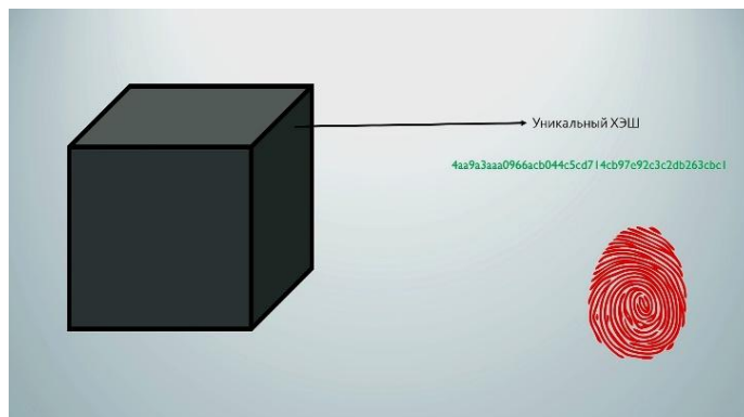
Рис. 1. Хэш блока
