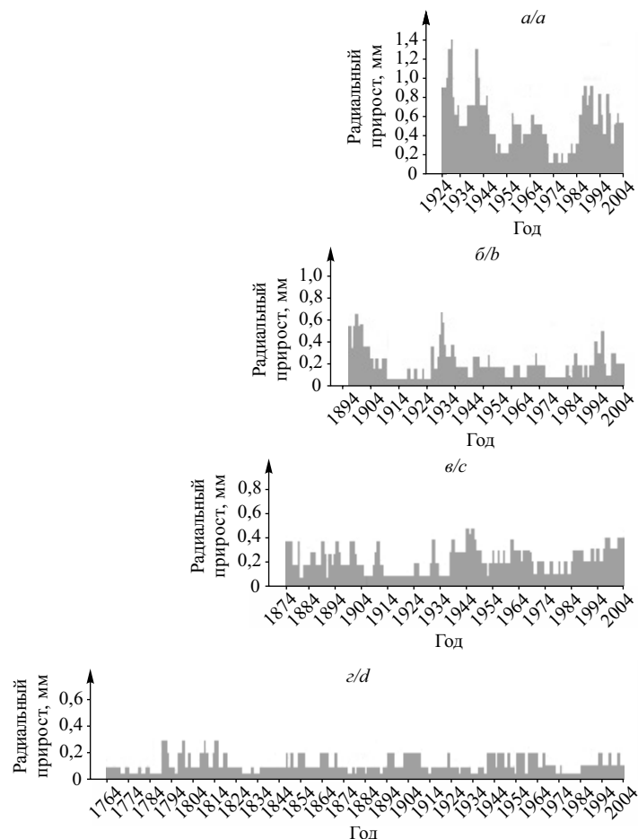
Рис. 1. Многолетний погодный ход изменчивости минимального индивидуального радиального прироста возрастных серий сосны на территории верхового болота Круки: а – 85 лет; б – 115 лет; в – 140 лет; г – 250 лет
