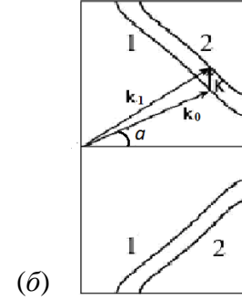
Рис. 1.(а) Схема квазиколлинейрной АО дифракции в ФК на сдвиговой SZ-УЗ волне (П(А) – поляризатор (анализатор), ПР – призма, ПП – пьезопреобразователь, ПГ – поглотитель, ФК – фотонный кристалл, a – длина ПП, l – длина АО взаимодействия); (б) диаграмма волновых векторов падающего (TE) и дифрагированного (TM) света при заданной частоте ( f_s ) ультразвука и длине волны ( \lambda ) света
