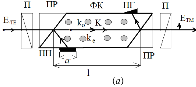
Рис. 1.(а) Схема квазиколлинейрной АО дифракции в ФК на сдвиговой SZ-УЗ волне (П(А) – поляризатор (анализатор), ПР – призма, ПП – пьезопреобразователь, ПГ – поглотитель, ФК – фотонный кристалл, a – длина ПП, l – длина АО взаимодействия); (б) диаграмма волновых векторов падающего (TE) и дифрагированного (TM) света при заданной частоте ( f_s ) ультразвука и длине волны ( \lambda ) света
