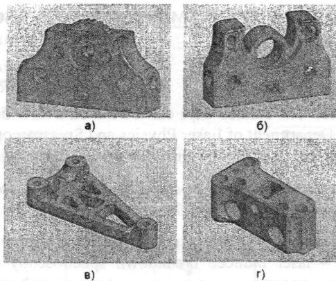
Рисунок 4 – Элементы столика: опоры для направляющих с ручным управлением перемещения (а); с возможностью закрепления мотора (б); предметная платформа с крепежами для держателей для предметного стекла (в); каретка одной из осей (г)
