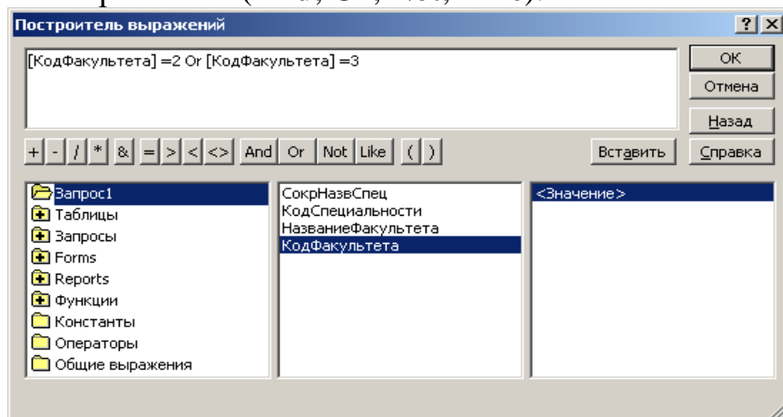
Рисунок 28. Пример критерия отбора, составленного в Построителе выражений
