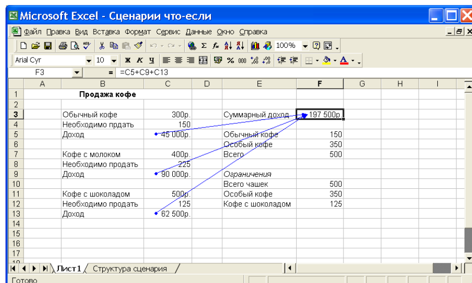
Рисунок 19. Постановка задачи
