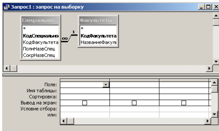
Рисунок 26. Окно Конструктора запроса с добавленными таблицами Специальности и Факультеты
