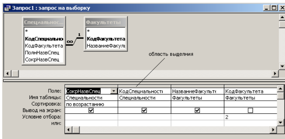
Рисунок 27. Пример запроса
