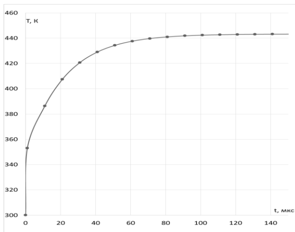
Рис. 1. Временная зависимость температуры в области пятна фокусировки ЛИ на поверхности пластины из титана в момент окончания воздействия излучения при энергии импульса E = 2 Дж
