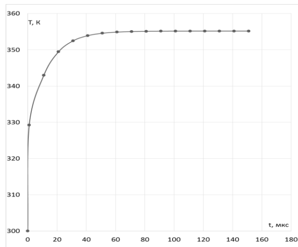
Рис. 2. Временная зависимость температуры в области пятна фокусировки ЛИ на поверхности пластины из кадмия в момент окончания воздействия излучения при энергии импульса E = 2 Дж
