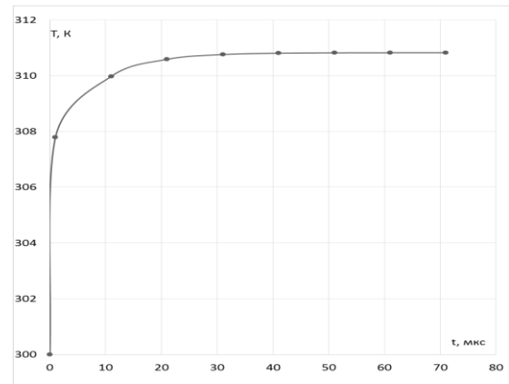
Рис. 3. Временная зависимость температуры в области пятна фокусировки ЛИ на поверхности пластины (медь) в момент окончания воздействия излучения из меди при энергии импульса E = 2 Дж
