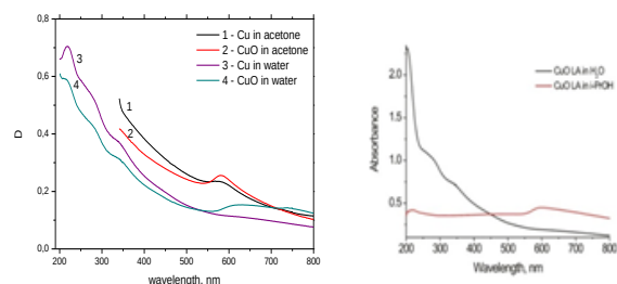
Рис. 3. Спектры поглощения НЧ, полученных ЛА в дистиллированной воде и ацетоне (слева) и в изопропиловом спирте (справа)
