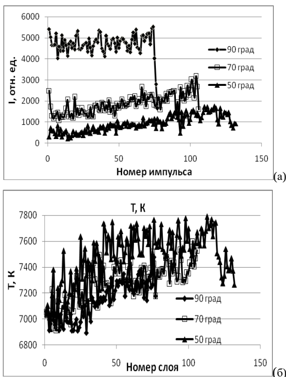
Рис. 1. Зависимости: а - интенсивности линии Cu (510.525 нм) и б - температуры от количества импульсов
