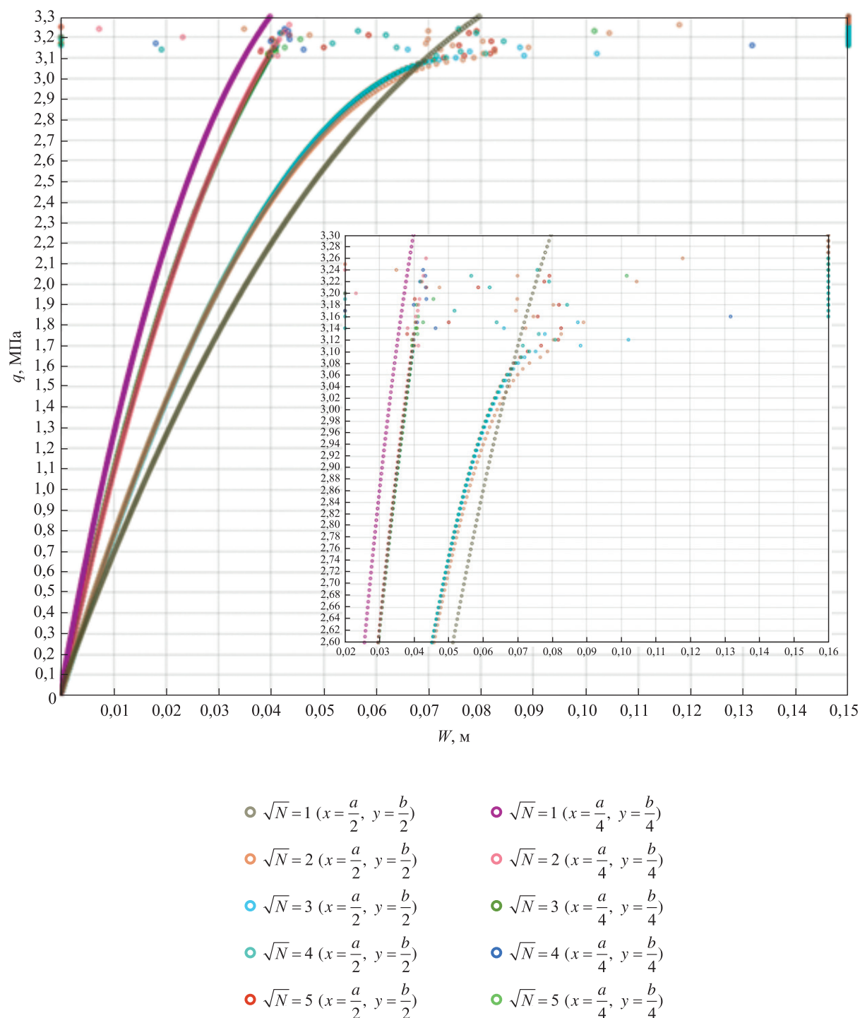
Рис. 7. График зависимости прогиба от нагрузки для конструкции без ребер
