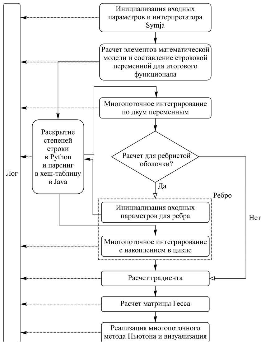
Рис. 3. Алгоритм моделирования
