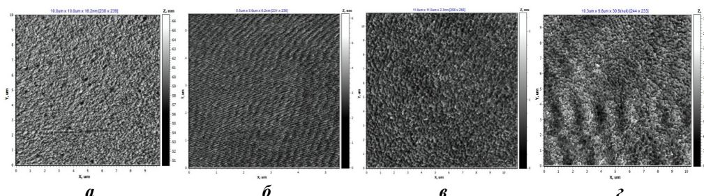
Рисунок 3. АСМ изображения поверхности структур V/Si 3 N 4 /Si: без отжига – ( а ), с отжигом при температуре 2000 °С – ( б ), 3000 °С – ( в ), 4000 °С – ( з )
