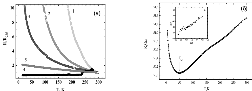
Рисунок 1. Температурные зависимости сопротивления пленок полиэтилентерефталата, имплантированных \text{Fe}^+ при плотности тока j = 4 \text{ мкА/см}^2 ; D, \text{ см}^{-2} : 1 – 2,5 \cdot 10^{16} ; 2 – 5 \cdot 10^{16} , 3 – 7,5 \cdot 10^{16} , 4 – 1 \cdot 10^{17} \text{см}^{-2} , 5 – 1,25 \cdot 10^{17} (a) и полиимида, имплантированного \text{Co}^+ D = 1,25 \cdot 10^{17} \text{ см}^{-2} , j = 12 \text{ мкА/см}^2 (б)
