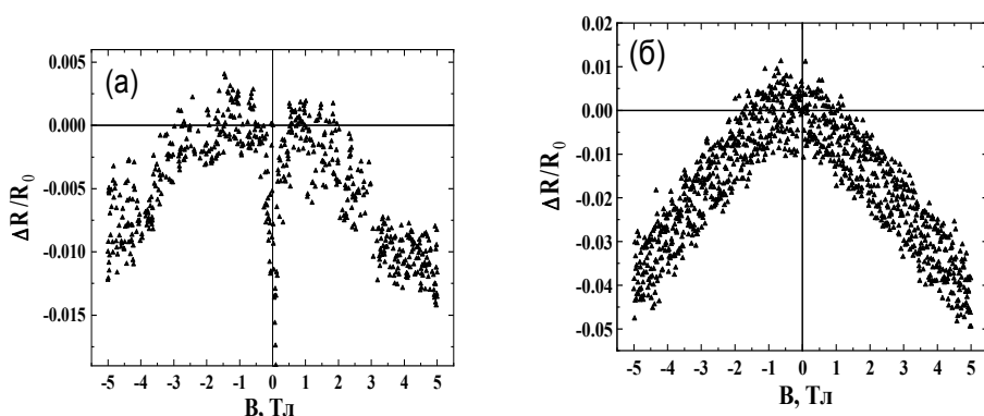
Рисунок 3. Магнитосопротивление пленки ПЭТФ, имплантированной \text{Fe}^+ , D = 7,5 \cdot 10^{16} \text{ см}^{-2} с диэлектрическим режимом переноса (а) и D = 1 \cdot 10^{17} \text{ см}^{-2} с металлическим режимом переноса (б) при T = 4,2 \text{ К} и j = 4 \text{ мкА/см}^2
