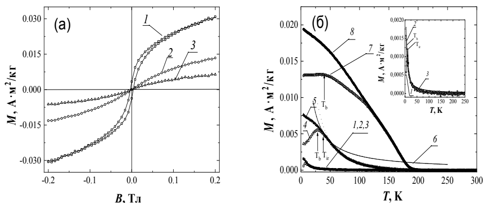
На вставке – температурная зависимость намагниченности для D = 5 \cdot 10^{16} \text{ см}^{-2} Рисунок 2. Петли гистерезиса намагниченности пленок полиимида, имплантированных \text{Co}^+ D = 5 \cdot 10^{16} \text{ см}^{-2} ; T, \text{ K} : 1 – 15; 2 – 100; 3 – 300 (а) и температурные зависимости намагниченности нанокластеров \text{Co}^+ при D, \text{ см}^{-2} : 5 \cdot 10^{16} (1, 2); 7,5 \cdot 10^{16} (4, 5); 1,25 \cdot 10^{17} (7, 8) (б).
