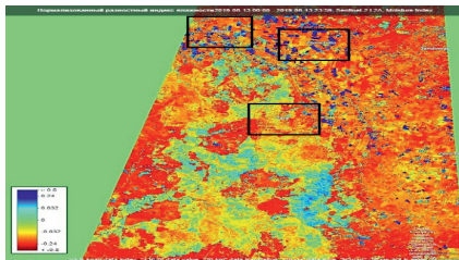
Рисунок 5 – NDMI после пожаров, 13.08.2019 г.
