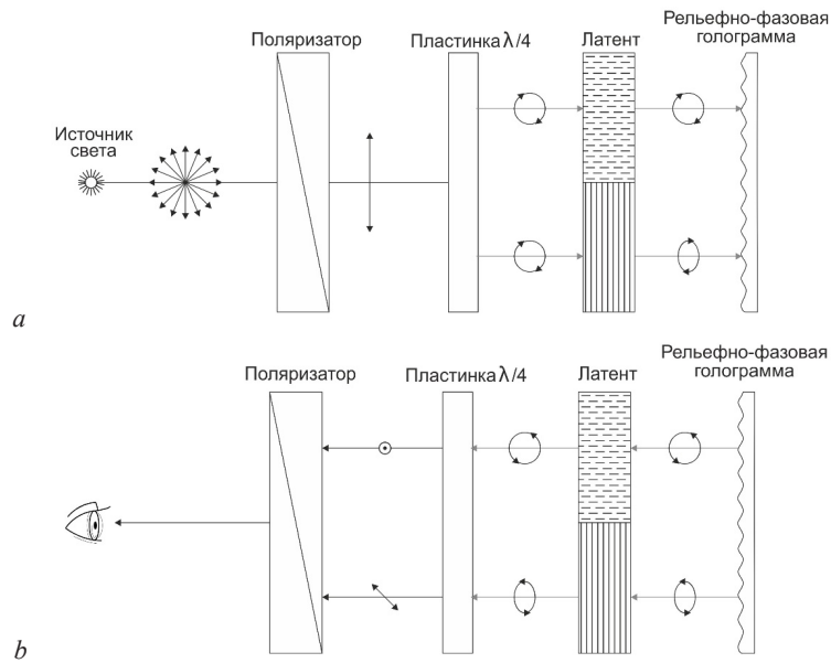
Рис. 2. Оптическая схема идентификации скрытого латентного изображения юниграммы: a – изменение поляризации излучения при прохождении слоев юниграммы до отражения от рельефо-фазовой голограммы; b – изменение поляризации излучения при прохождении слоев юниграммы после отражения от рельефо-фазовой голограммы
