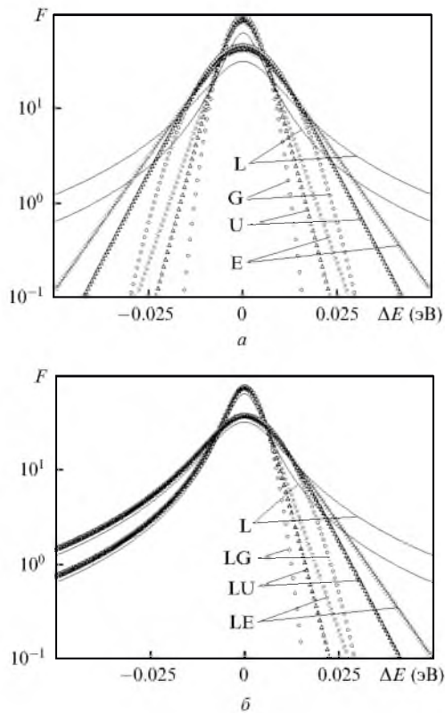
Рис.1. Спектральные распределения симметричных (а) и несимметричных (б) контуров уширения линии излучения для параметра уширения \gamma_L = 5 и 10 мэВ.
