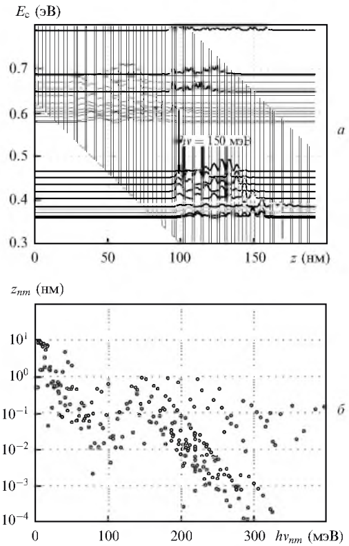
Рис.2. Диаграмма зоны проводимости E_c(z) и квадраты модулей волновых функций электронов (а) и дипольные матричные элементы переходов z_{nm} (б) для квантово-каскадной структуры Al 0.48 In 0.52 As – Ga 0.47 In 0.53 As в электрическом поле с напряженностью E = 3.25 \times 10^4 \text{ В/см} ; h\nu_{nm} = E_n - E_m .
