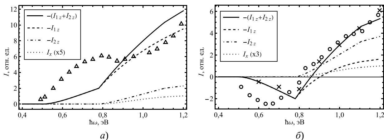
Рис. 2. – Зависимости компонент фототока от энергии фотонов при возбуждении гетероструктуры слева (а) и справа (б). Крестики соответствуют результатам моделирования методом Монте-Карло, треугольники и кружки – экспериментальным данным.
