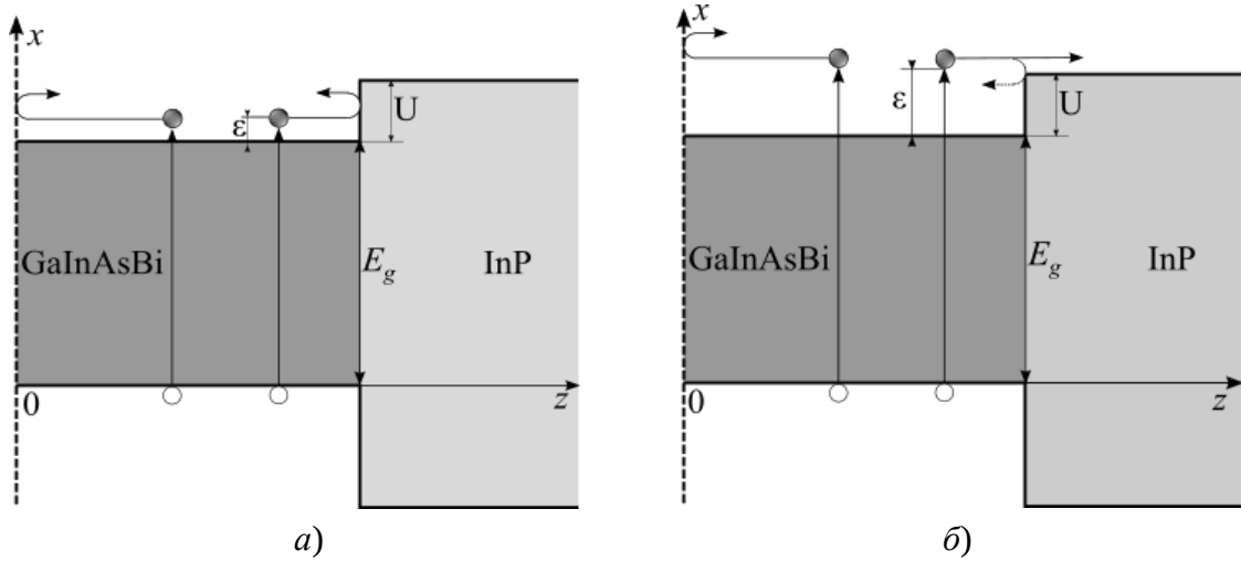
Рис. 1. – Энергетические диаграммы гетероперехода при полном (а) и частичном (б) отражении электронов от потенциального барьера. Штриховая стрелка означает прекращение отражения когда \varepsilon > U/(1-m_1/m_2) .
