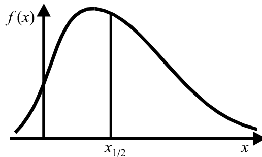
Рис. 6. Медиана распределения.
