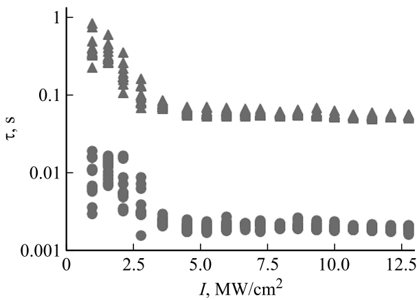
Рис. 4. Зависимость времени релаксации ловушечных уровней от интенсивности падающего излучения.
