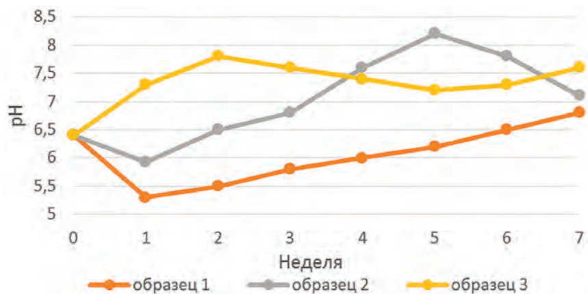
Рисунок 2 – Динамика изменения рН среды компостируемой смеси
