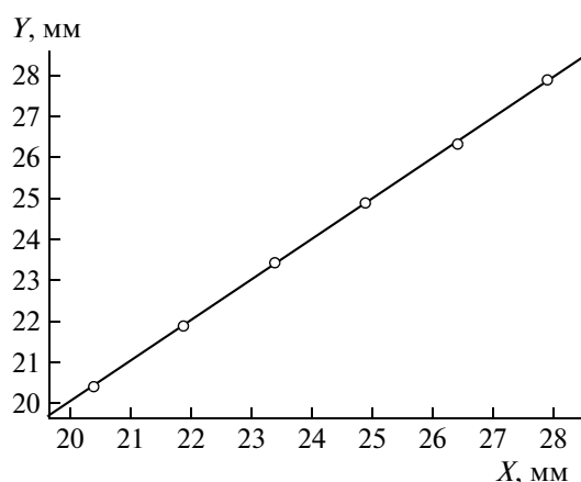
Рис. 3. Установленное положение радиоактивного источника ( X ) и измеренное ( Y ) при напряжении на анодной проволоочке 3.4 кВ.
