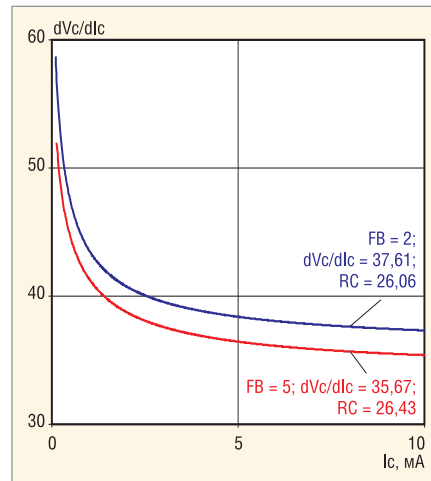
Рис. 19. Зависимость производной от коллекторного напряжения по коллекторному току от коллекторного тока для БТ с ОЗ в насыщении при \text{FB} = 2 и \text{FB} = 5
