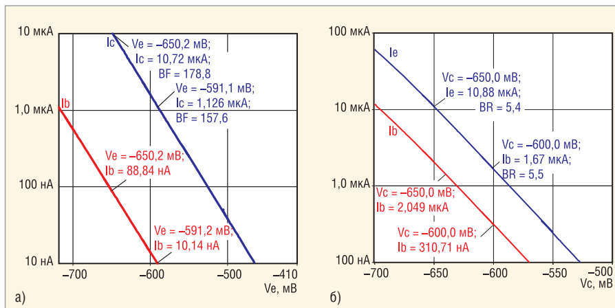
Рис. 11. Область характеристик Гумеля с одинаковым наклоном кривых
