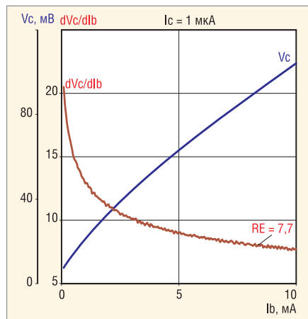
Рис. 16. Результаты измерений выходной характеристики БТ с разомкнутым коллектором
