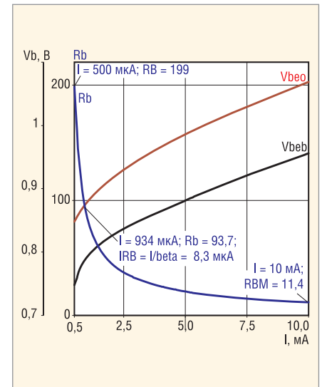
Рис. 21. Результаты измерений диодной характеристики эмиттерного перехода
