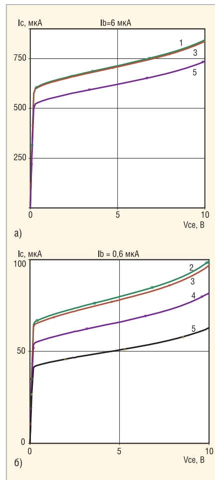
Рис. 8. Выходные характеристики БТ в схеме с ОЭ
