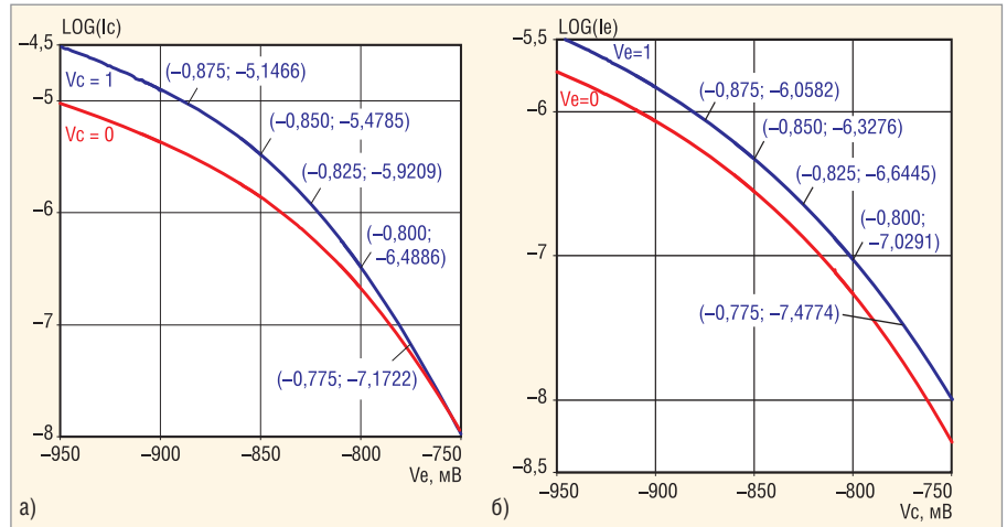
Рис. 14. Зависимость \ln I_C от напряжения на эмиттере V_E при V_B = 0 в режиме высокого уровня инжекции а) для прямого включения БТ, б) для инверсного включения БТ
