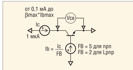
Рис. 18. Схема включения для измерения выходной характеристики БТ с ОЗ в насыщении
