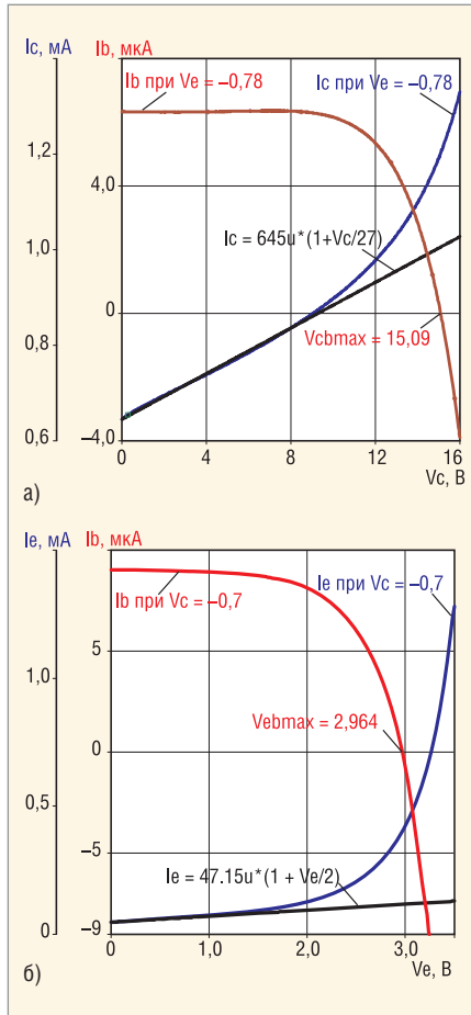
Рис. 7. Характеристики Эрли
