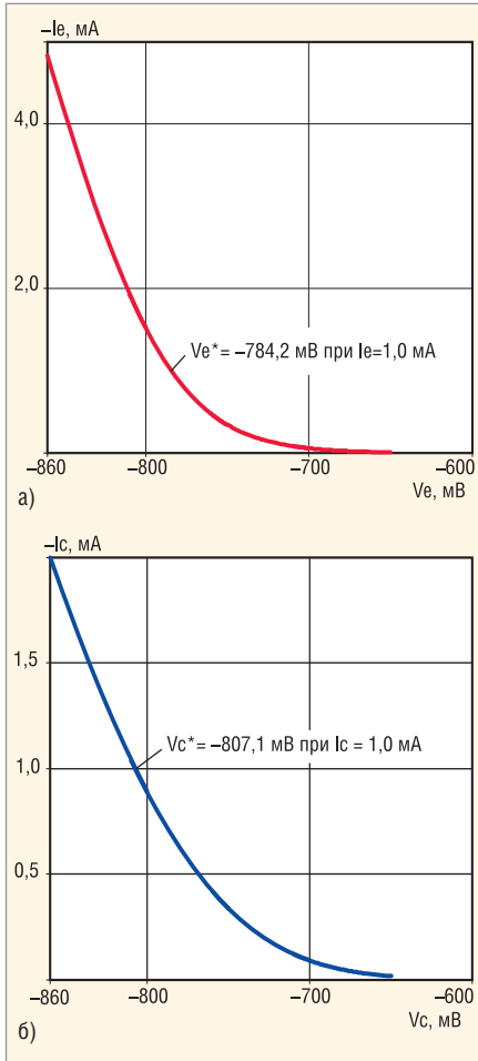
Рис. 5. Входная характеристика БТ с ОБ
