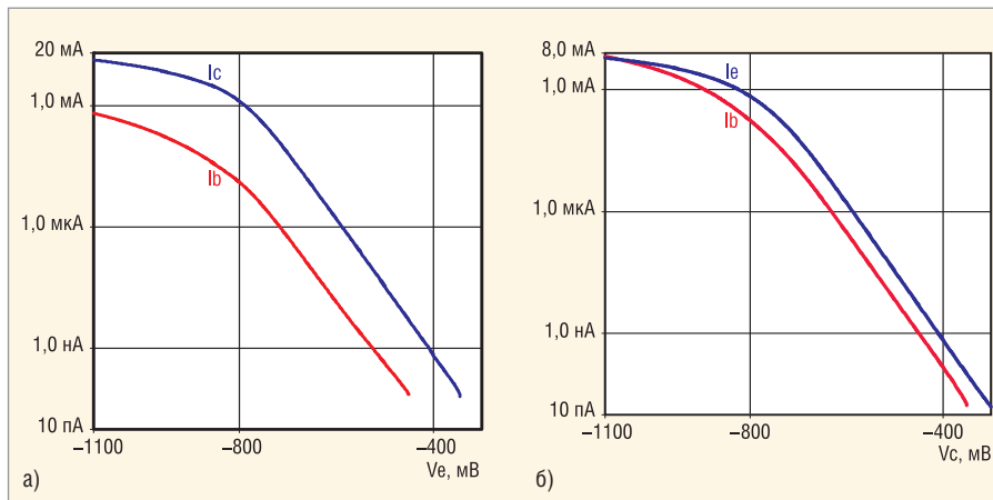
Рис. 10. Характеристики Гумеля
