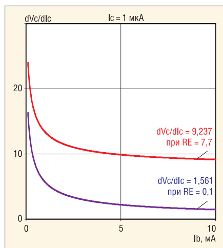
Рис. 17. Результаты моделирования выходной характеристики БТ с разомкнутым коллектором при различной величине параметра RE
