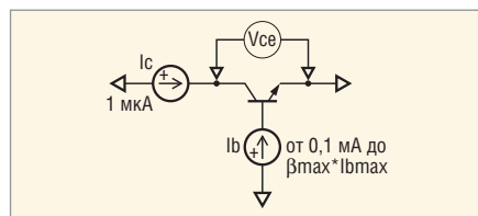
Рис. 15. Схема включения для измерения выходной характеристики БТ с разомкнутым коллектором
