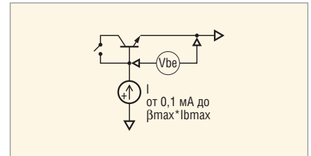
Рис. 20. Схема включения БТ для измерения диодной характеристики эмиттерного перехода
