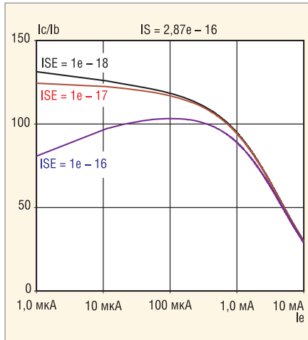
Рис. 13. Результаты моделирования зависимости \beta = \beta(I_E) при разной величине ISE
