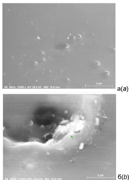
Рис. 4. Поверхность пленок ПЭТФ, облученных ионами фосфора с дозами: а) 200 мкКл; б) 2000 мкКл
