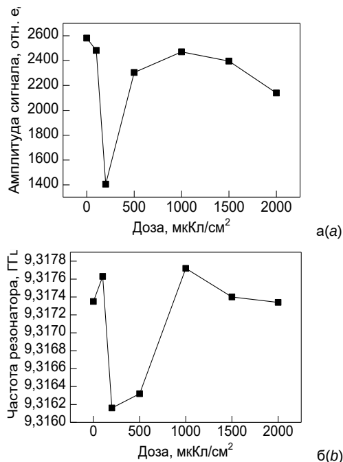
Рис. 2. Зависимость амплитуды сигнала ЭПР эталона рубина (а) и частоты резонатора (б) от дозы облучения ионами фосфора пленок ПЭТФ
