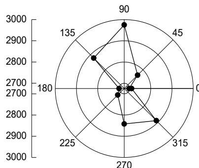
Рис. 3. Угловая зависимость амплитуды сигнала ЭПР в пленке ПЭТФ, облученной ионами фосфора с дозой 200 мкКл/см 2
