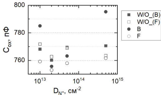
Рисунок 2 – Зависимость величины емкости подзатворного окисла транзистора ( C_{ox} ) от дозы имплантированного азота ( D_{N^+} , см -2 ) при прямом (F) и обратном (B) порядке термообработки для образцов, имплантированных N + , и контрольных образцов (W/O)
