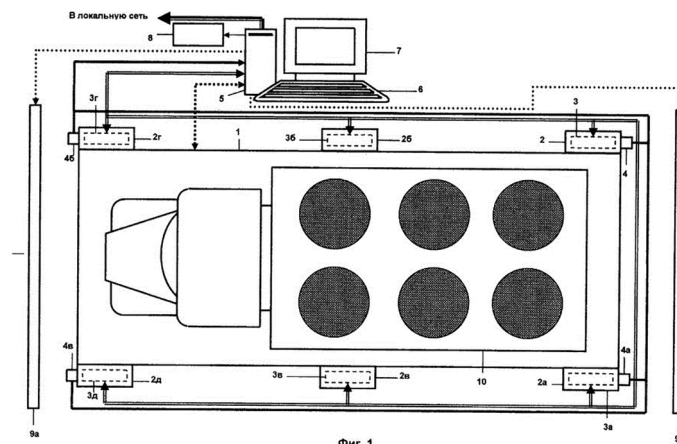
Рисунок 2 – Транспортный радиационный портальный монитор
