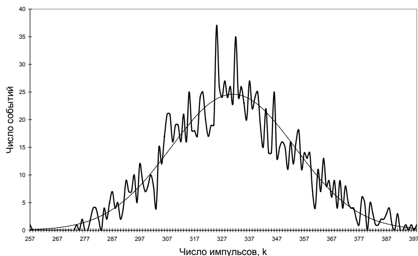
Рис. 2. ВР для объема выборки N = 1400
