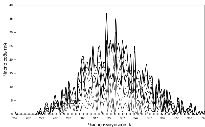
Рис. 3. Графики функций ВР^1 \div ВР^7
