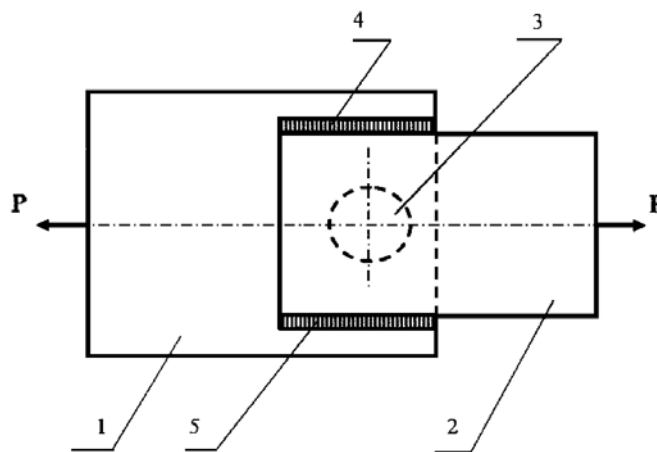
Рис. 1. Нахлесточное сварное соединение с продольными угловыми швами дополненное сварной точкой: 1 и 2 – соединяемые детали, 3 сварная точка, 4,5 – угловые сварные швы, P – рабочая нагрузка
